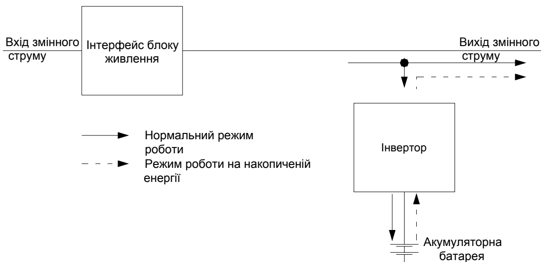
Рисунок В.3 – Робота АБП у лінійному інтерактивному режимі
