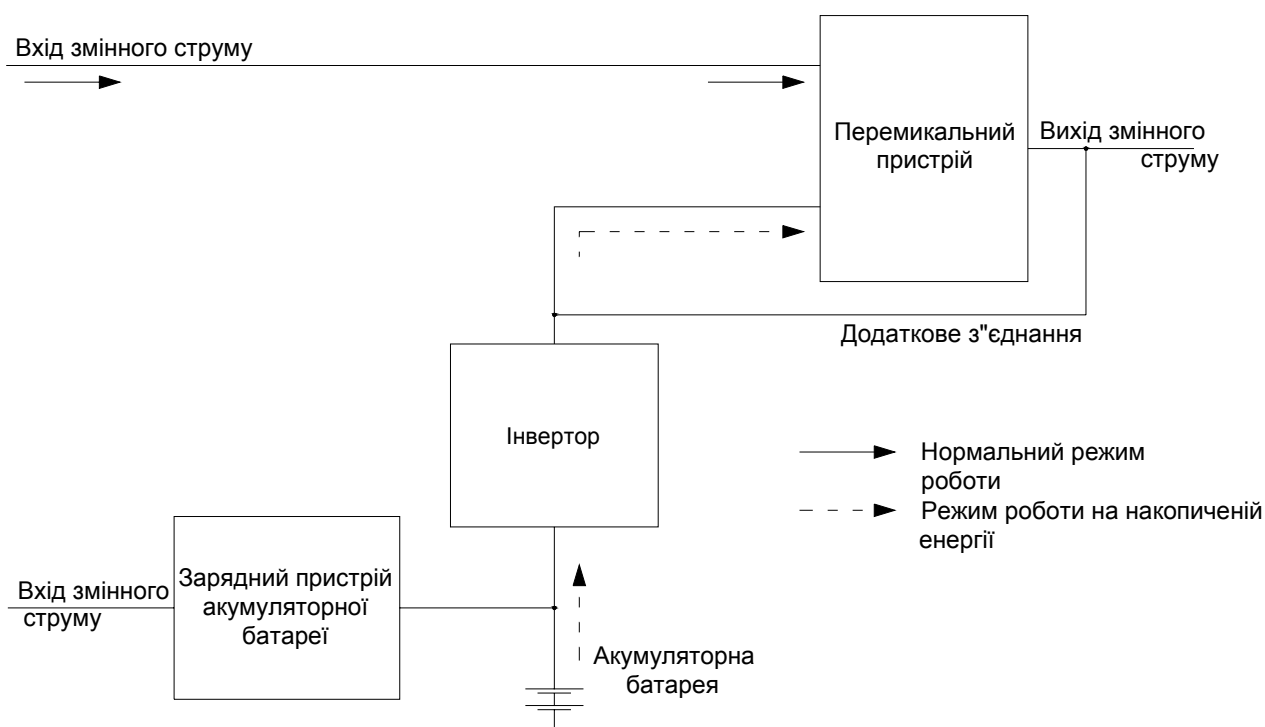
Рисунок В.5 – Схема пасивної роботи АБЖ із виділеним резервом
