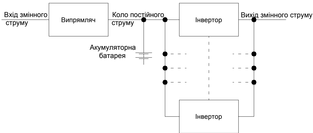
Рисунок А.5а – Частково паралельний АБЖ (із паралельним інвертором)
