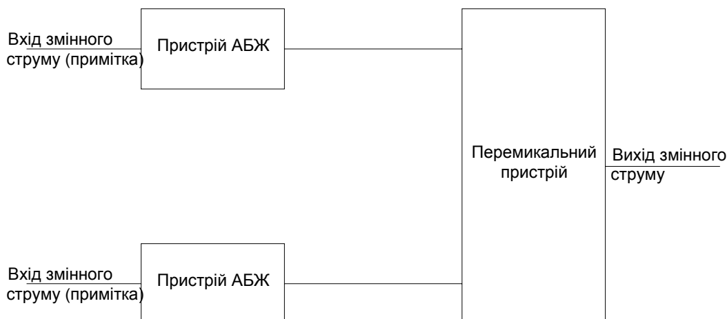
Рисунок А.6 – АБЖ із виділенням резервом без обвідного кола
