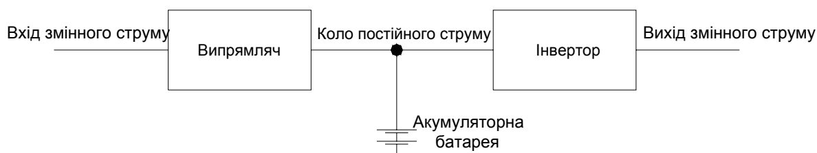
Рисунок А.1 – Одиночний АБЖ із загальним для інвертора та акумуляторної батареї випрямлячем
