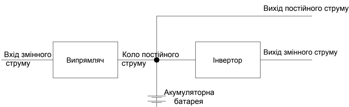
Рисунок А.3 – Одиночний АБЖ із виходами змінного та постійного струму
