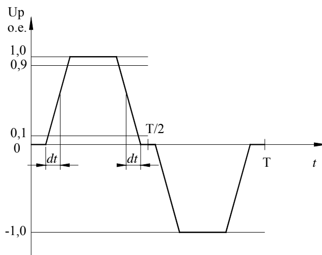
Рисунок 4 - Приклад сигналу несинусоїдальної вихідної напруги
