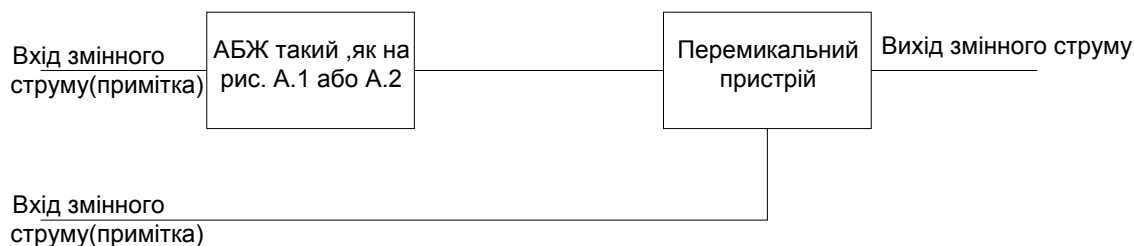
Рисунок А.4 – Одиночний АБЖ з обвідним колом
