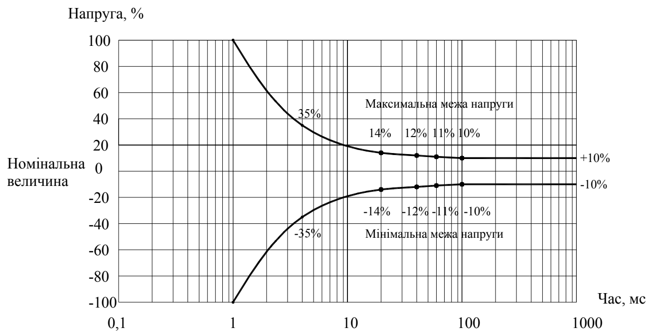
Рисунок 1 - Класифікація 1 вихідних динамічних робочих характеристик
